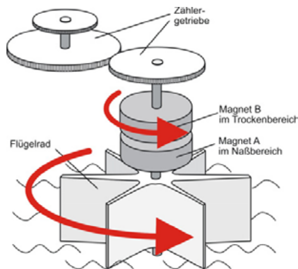
Eine zu schnelle und ruckartige Wasserströmung führt zu einem Abriss der Magnetkupplung im Wasserzähler.
